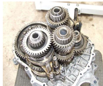
Reparacion de engranaje
